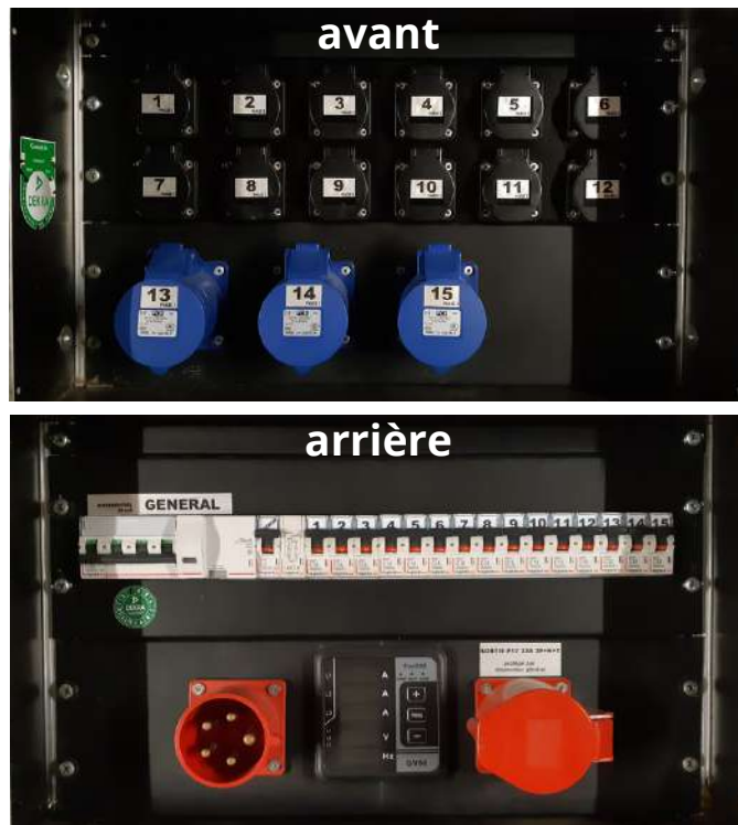
Armoire électrique (Flight) P17-32A
