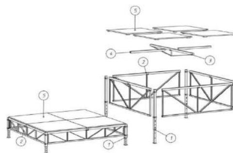
STACCO / Scène Trad
